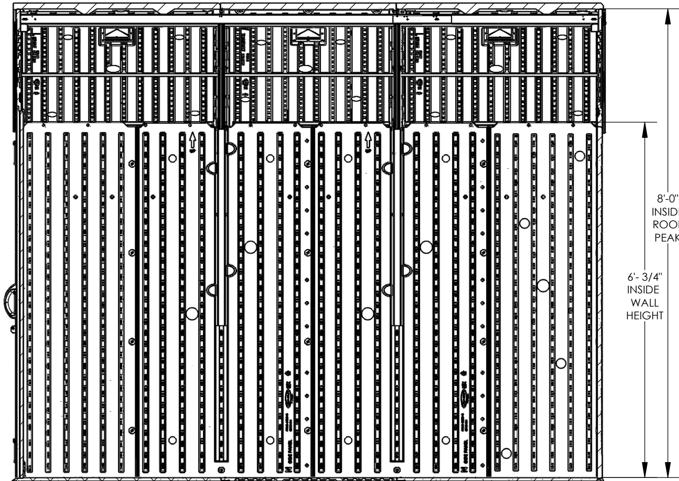
SECTION A-A
