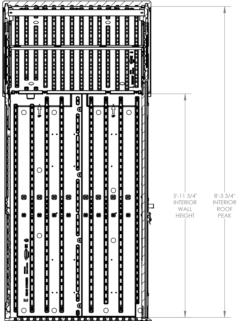
SECTION A-A SCALE 1 : 16
